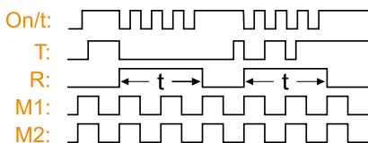
Временная диаграмма и поведение светодиодов
