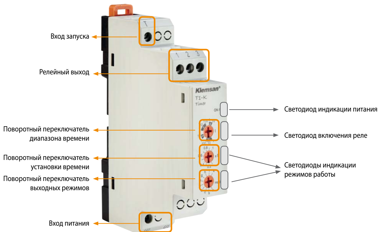
Многофункциональный таймер T1-K
