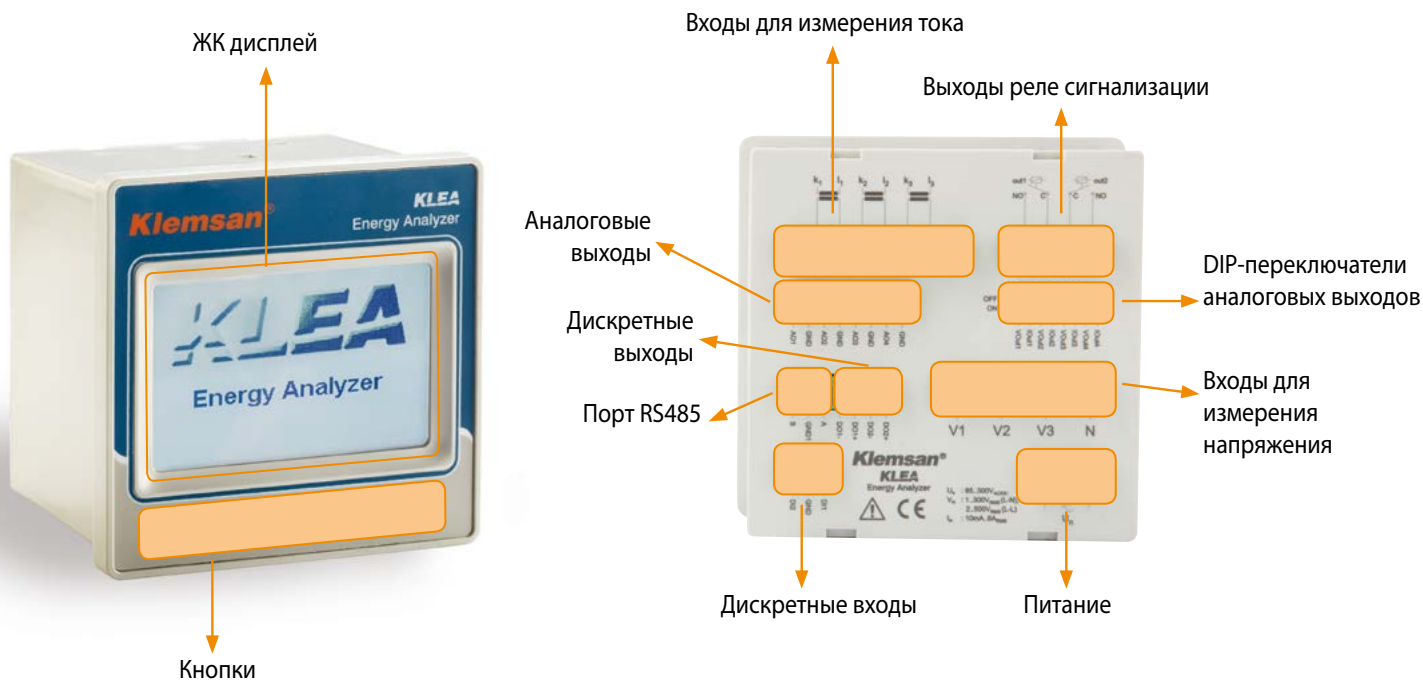
Анализатор электроэнергии KLEA 324P
